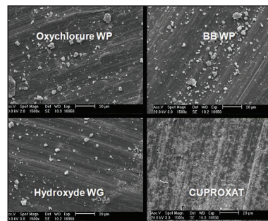
Couverture du végétal par les particules de cuivre (microscope électronique)
