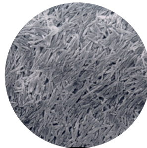
Grossissement x 3000 Tri-Base Flow appliqué sur feuille (Microscope électronique)
